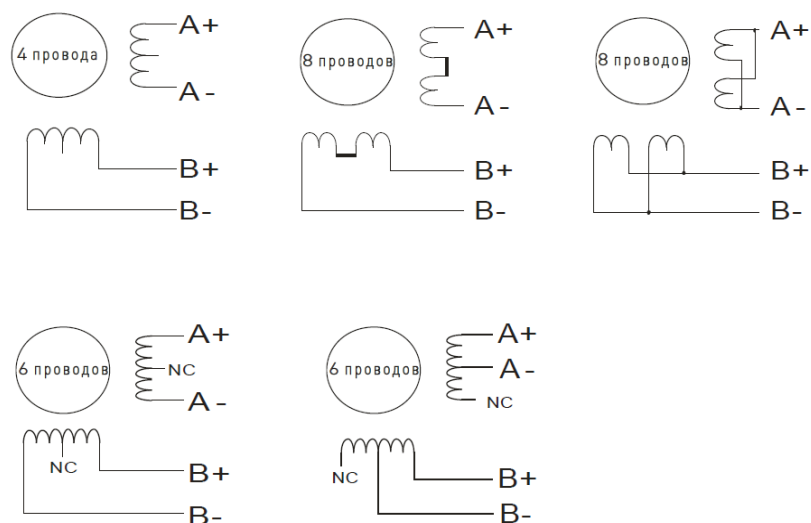
Рисунок 3 — Схема подключения двигателей с 4, 6 и 8 проводами.
