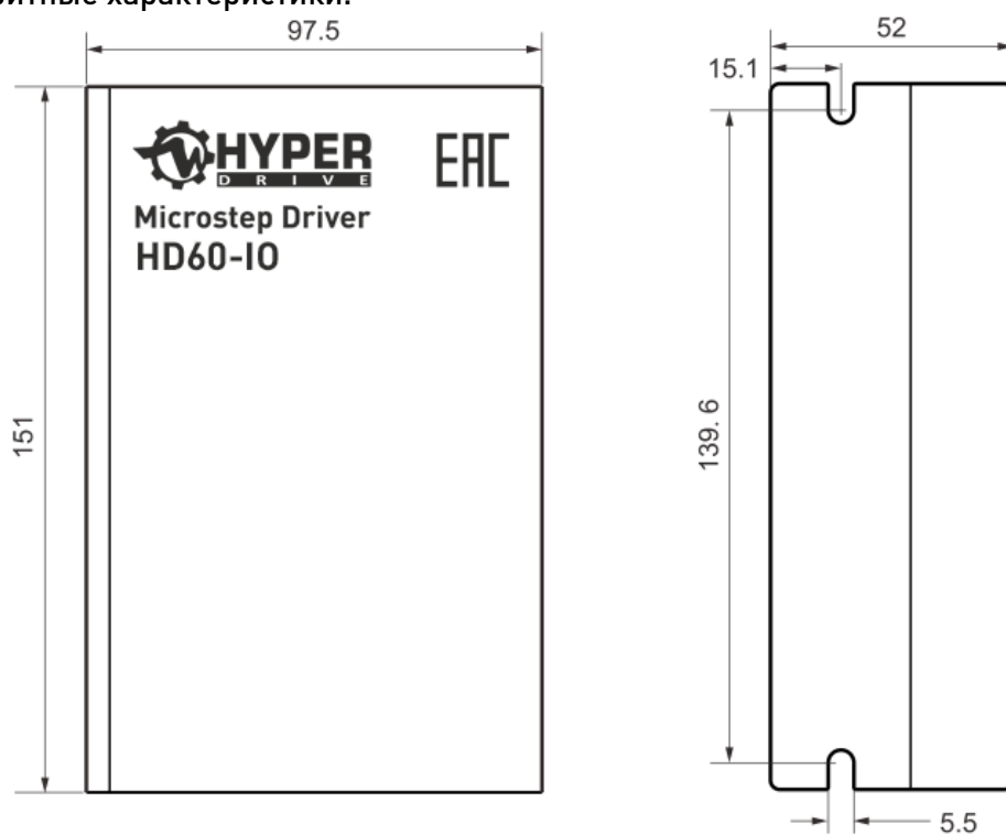
Рисунок 1 — Габаритные характеристики драйвера.
