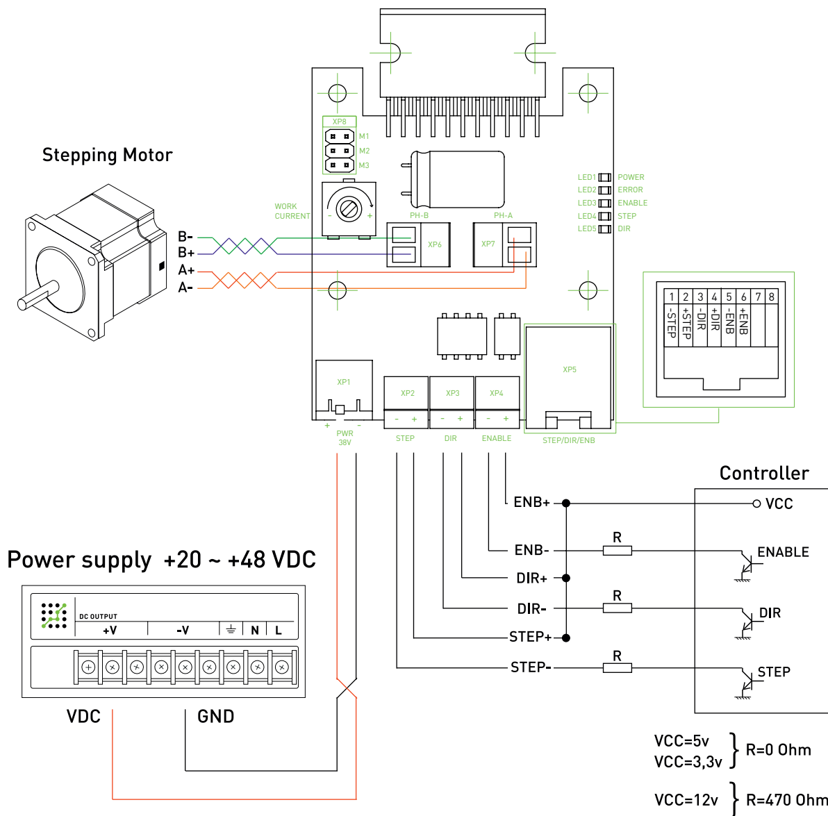
Рис. 2. Схема подключения драйвера ШД
