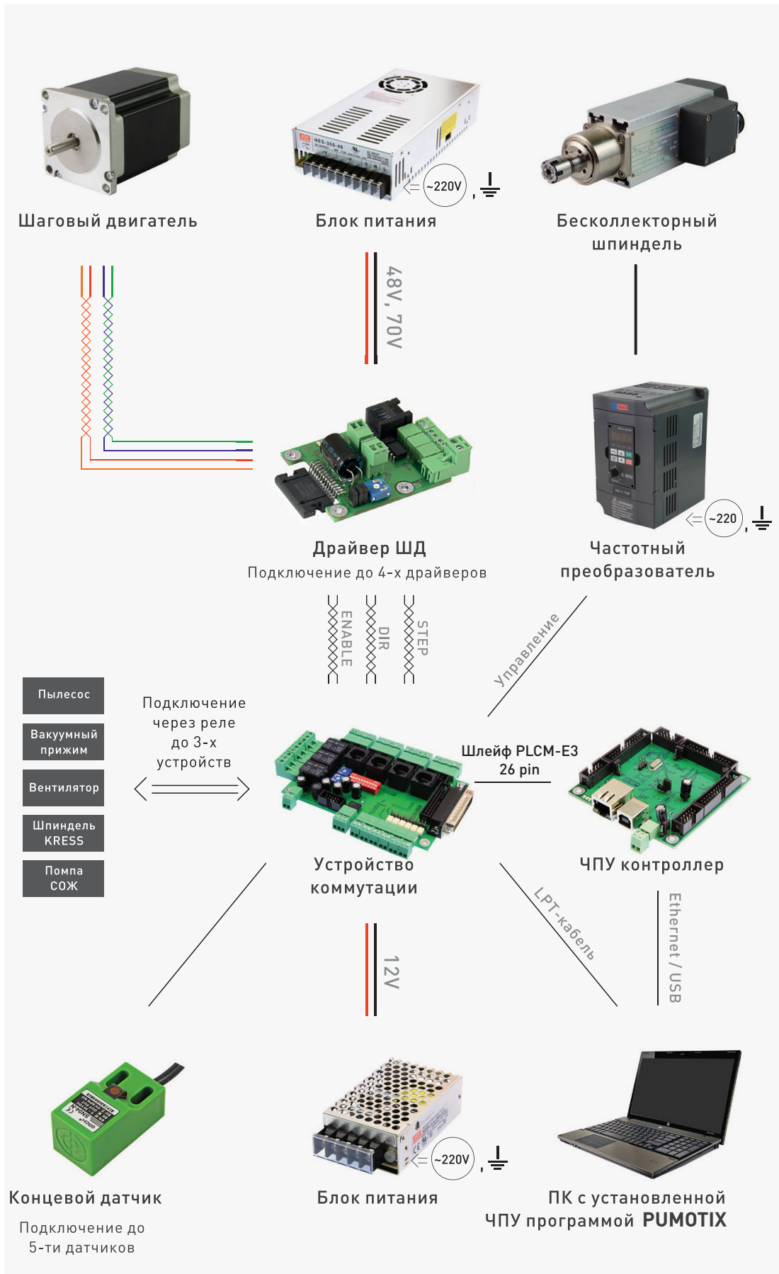
Рис. 3. Общая схема системы управления станком ЧПУ
