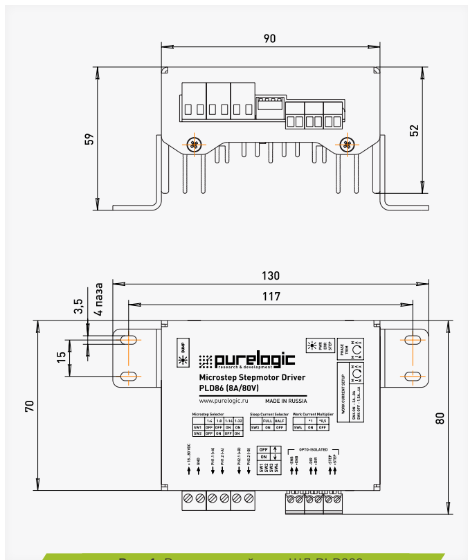
Рис. 1. Размеры драйвера ШД PLD330
