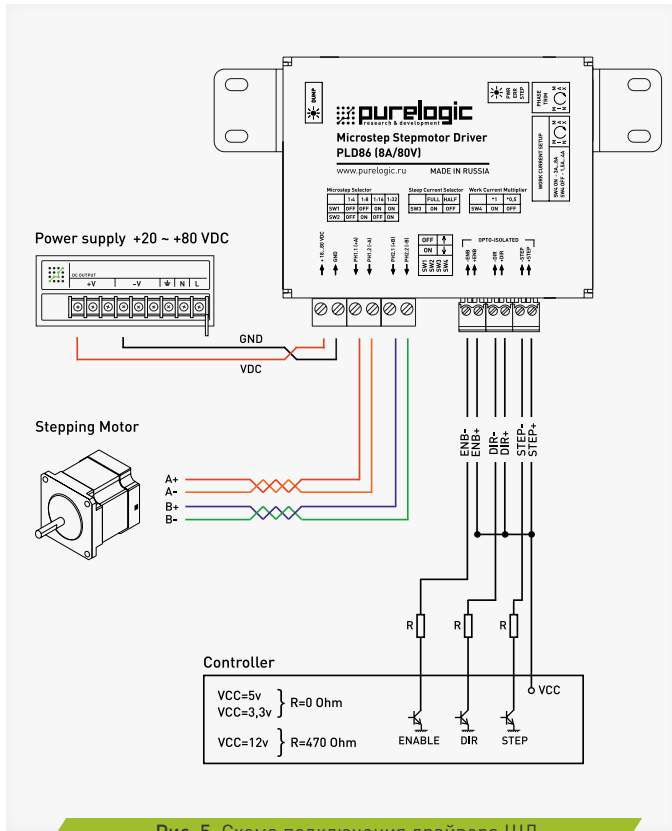
Рис. 5. Схема подключения драйвера ШД
