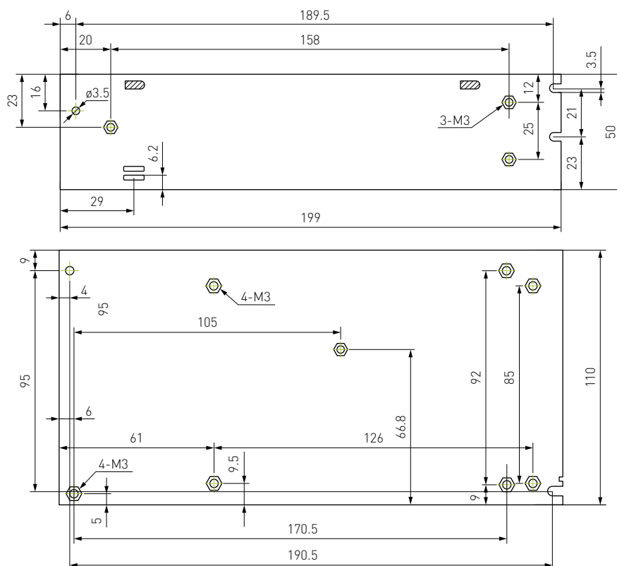
Рисунок 2 – Габаритный чертеж источника питания LSP-260-24.
