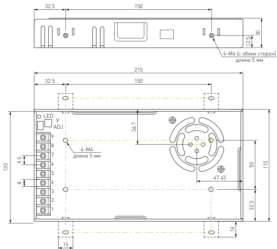
Рисунок 3 – Габаритный чертеж источников питания LSP-360-36, LSP-360-48, LSP-400-60.
