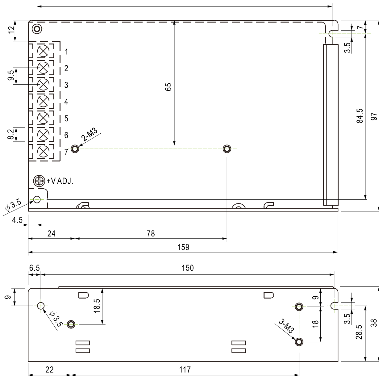
Рисунок 2 – Габаритные и присоединительные размеры источника питания GD-60-12-24.
