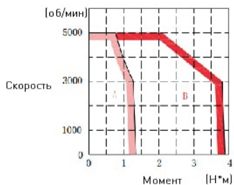
Кривая момента-скорости
