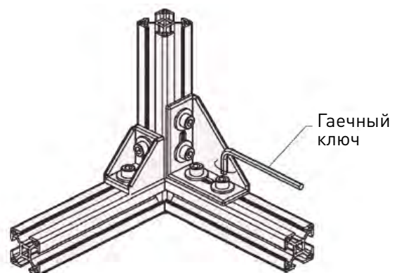
Схема сборки
