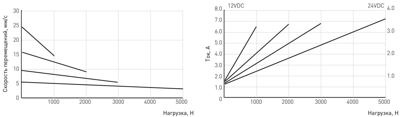
Рисунок 3 – Результаты испытаний актуаторов TGB.
