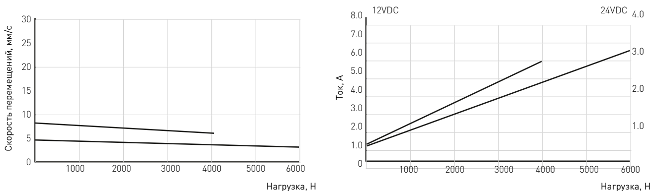
Рисунок 4 – Результаты испытаний актуаторов TGB-L.
