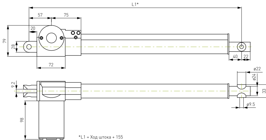
Рисунок 1 – Габаритные и присоединительные размеры (мм) актуаторов TGB.
