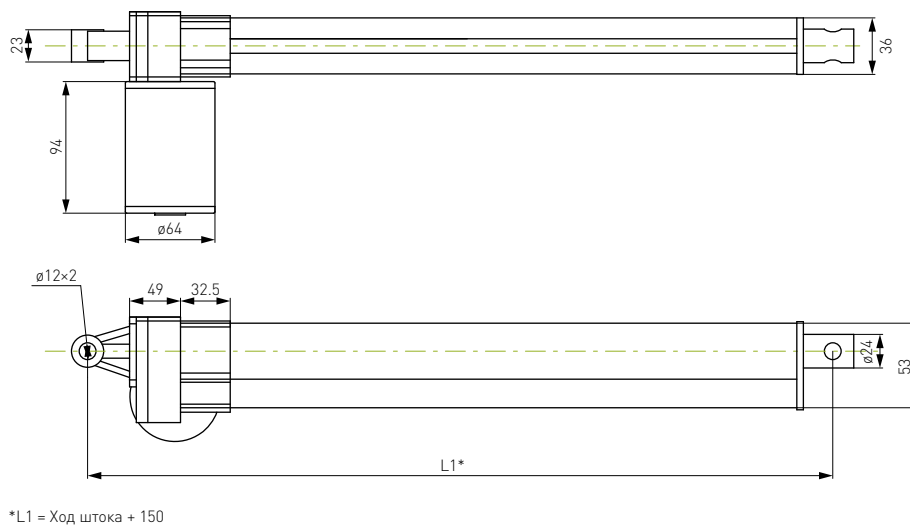
Рисунок 2 – Габаритные и присоединительные размеры (мм) актуаторов TGB-L.
