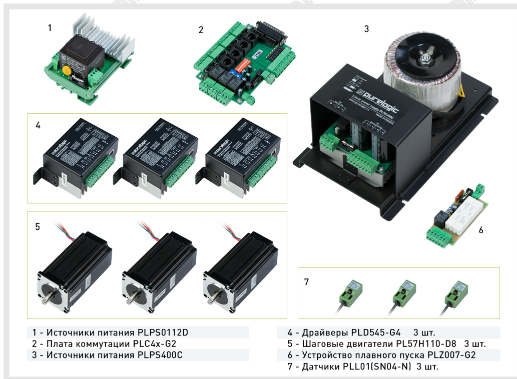
Рис. 1 Наборы PLD545-G4-S1L. Управление по интерфейсу LPT. Схема подключения набора показана на странице 2.
