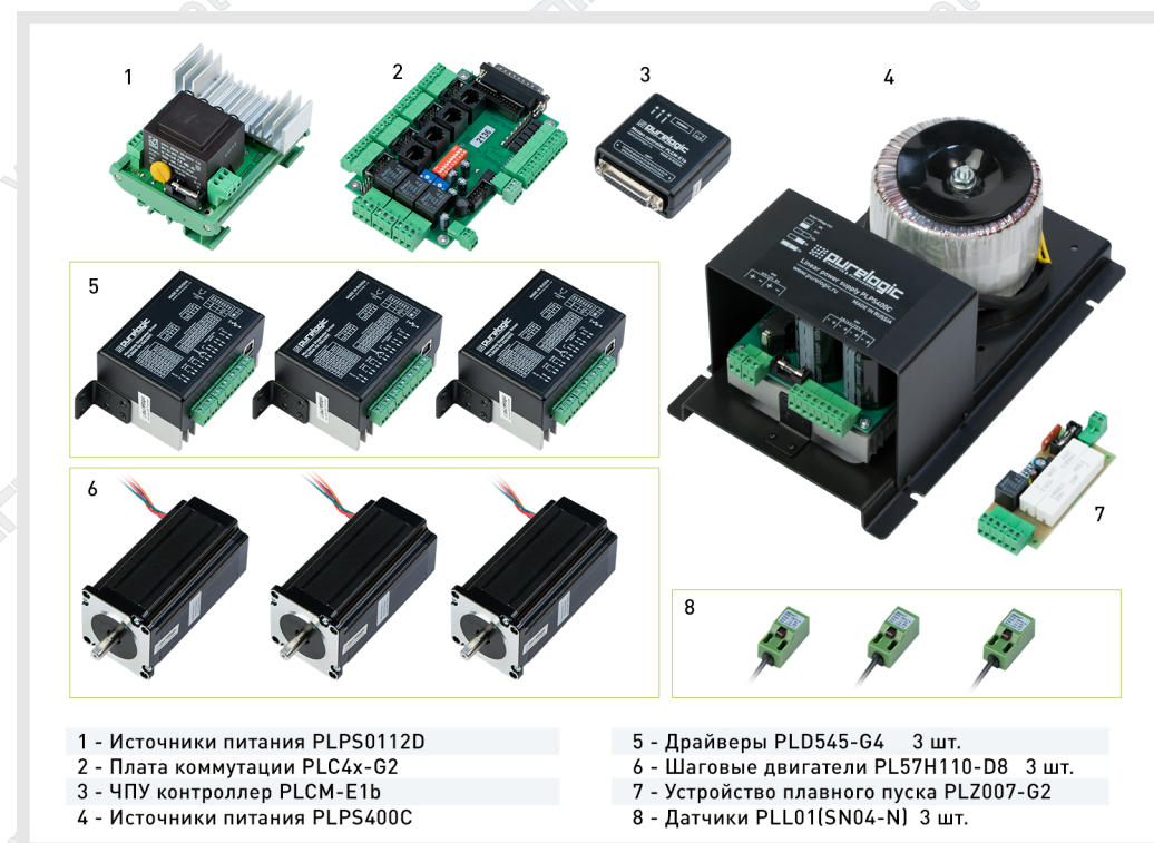
Рис. 2 Наборы PLD545-G4-S1E. Управление по интерфейсу Ethernet. Схема подключения набора показана на странице 3.
