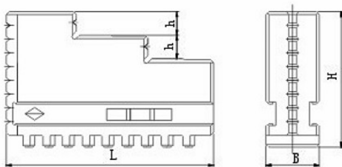
Рис. 2. Габаритные и установочные размеры изделия
