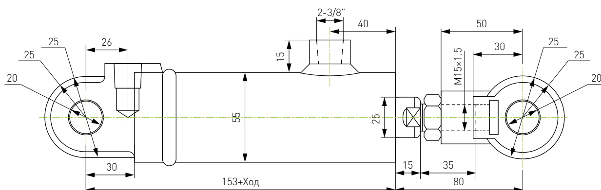
Рисунок 1 – Геометрические размеры (мм).
