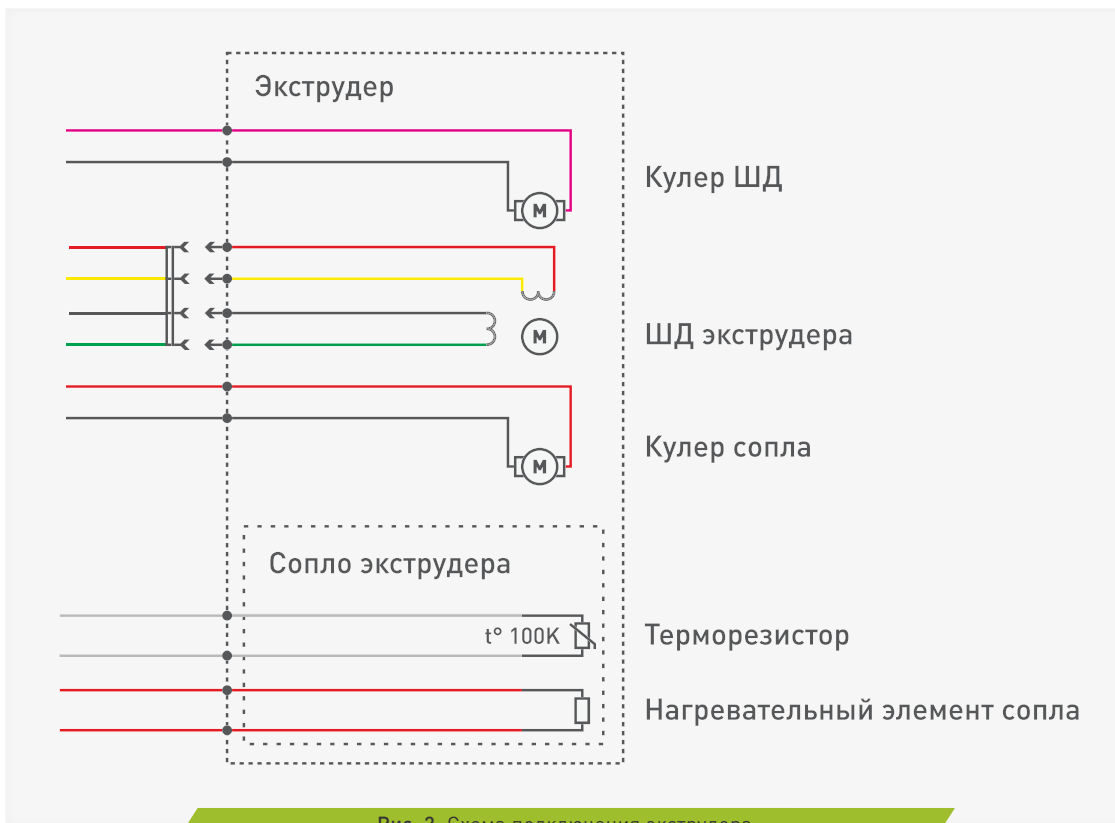
Рис. 2. Схема подключения экструдера
