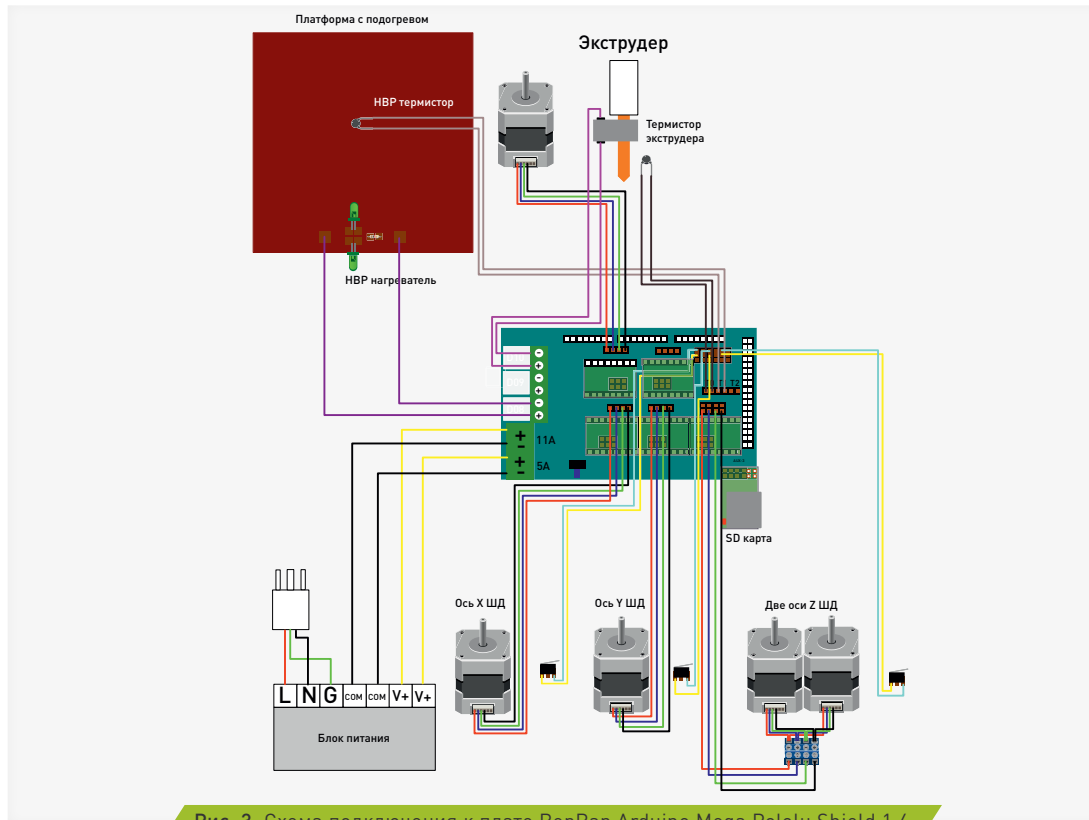
Рис. 3. Схема подключения к плате RepRap Arduino Mega Pololu Shield 1.4
