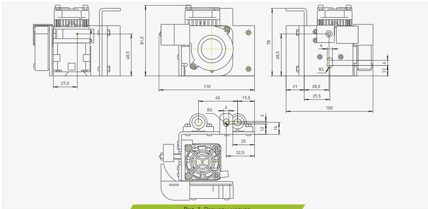
Рис. 1. Размеры модуля
