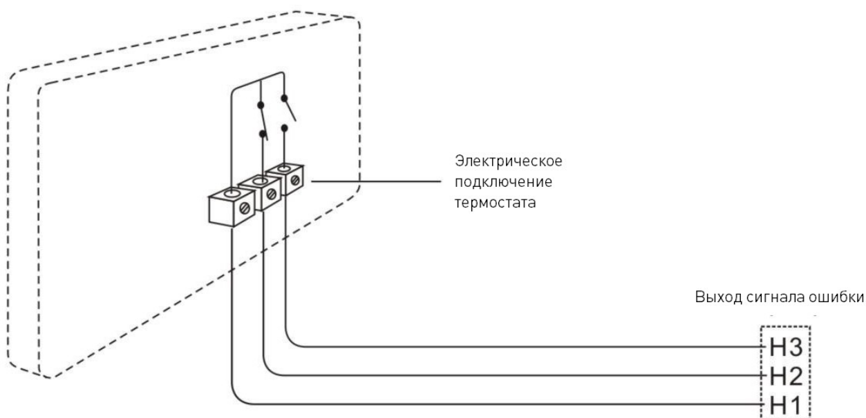
Рисунок 6 – Схема подключения выходов сигнала ошибки (чиллеры 220 В).
