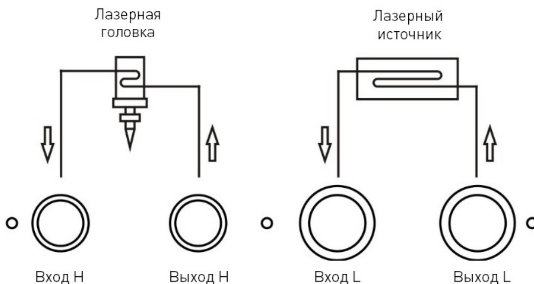
Рисунок 3 – Способ соединения чиллера и лазерного станка.
