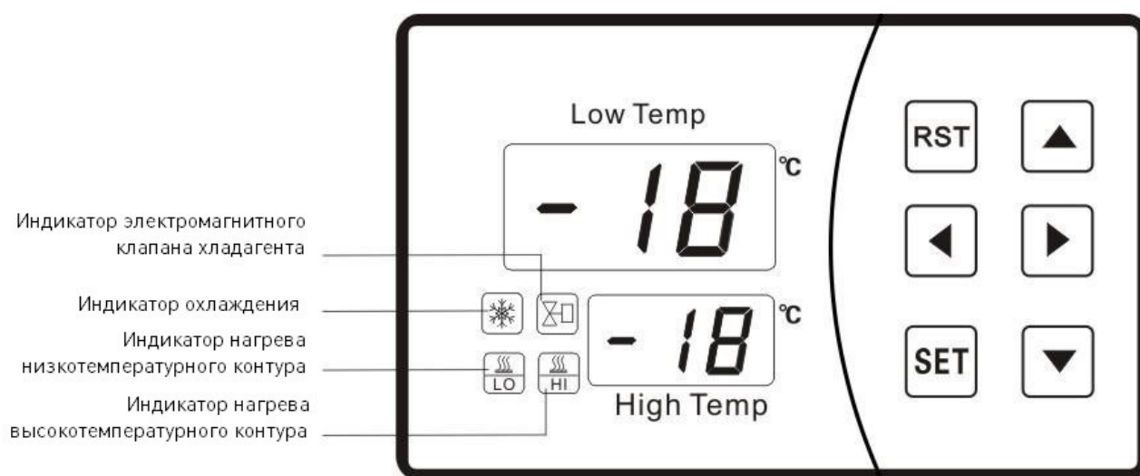
Рисунок 4 – Панель контроллера температуры чиллеров S&A CWFL (220 В).
