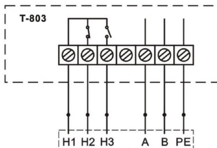
Рисунок 7 – Схема подключения выходов сигнала ошибки и интерфейса MODBUS RS-485 (чиллеры 380 В).
