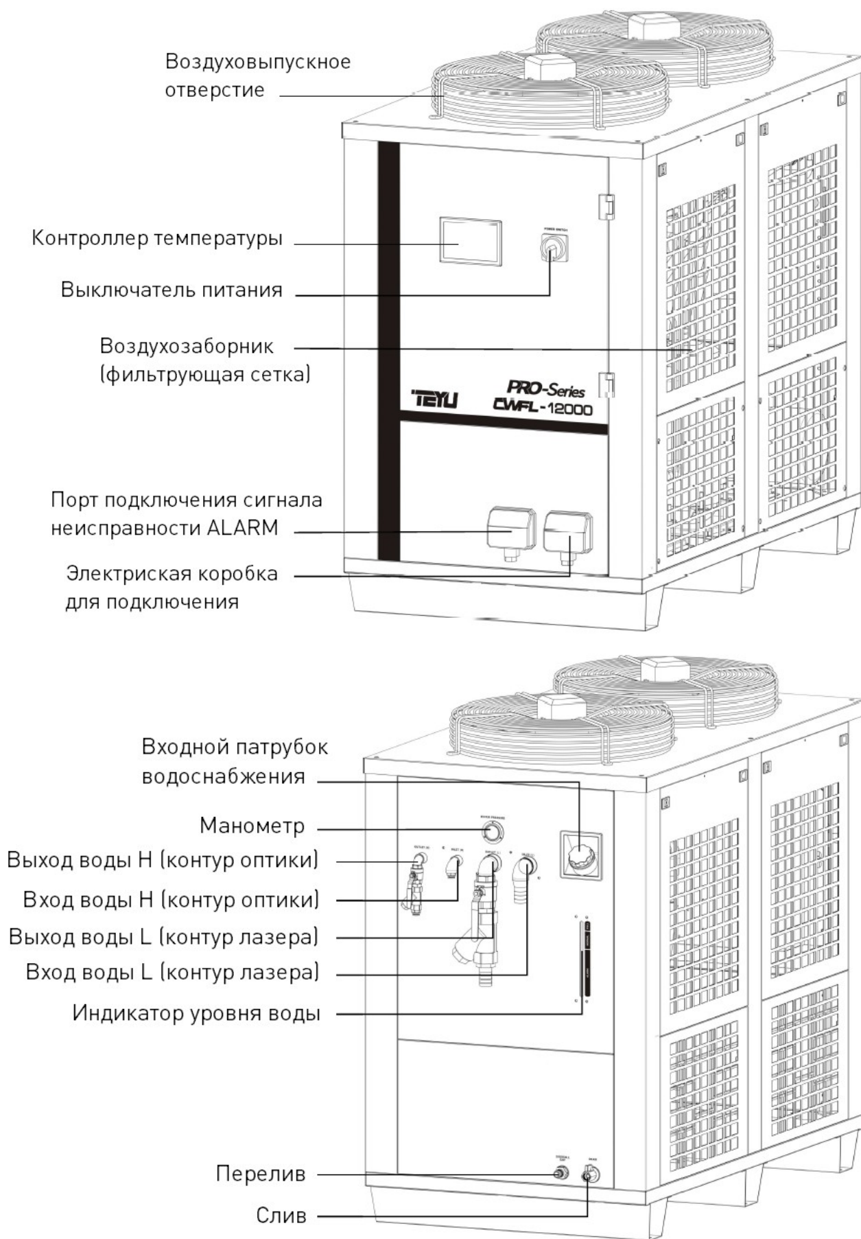
Рисунок 2 – Элементы чиллеров для лазеров от 12 кВт.
