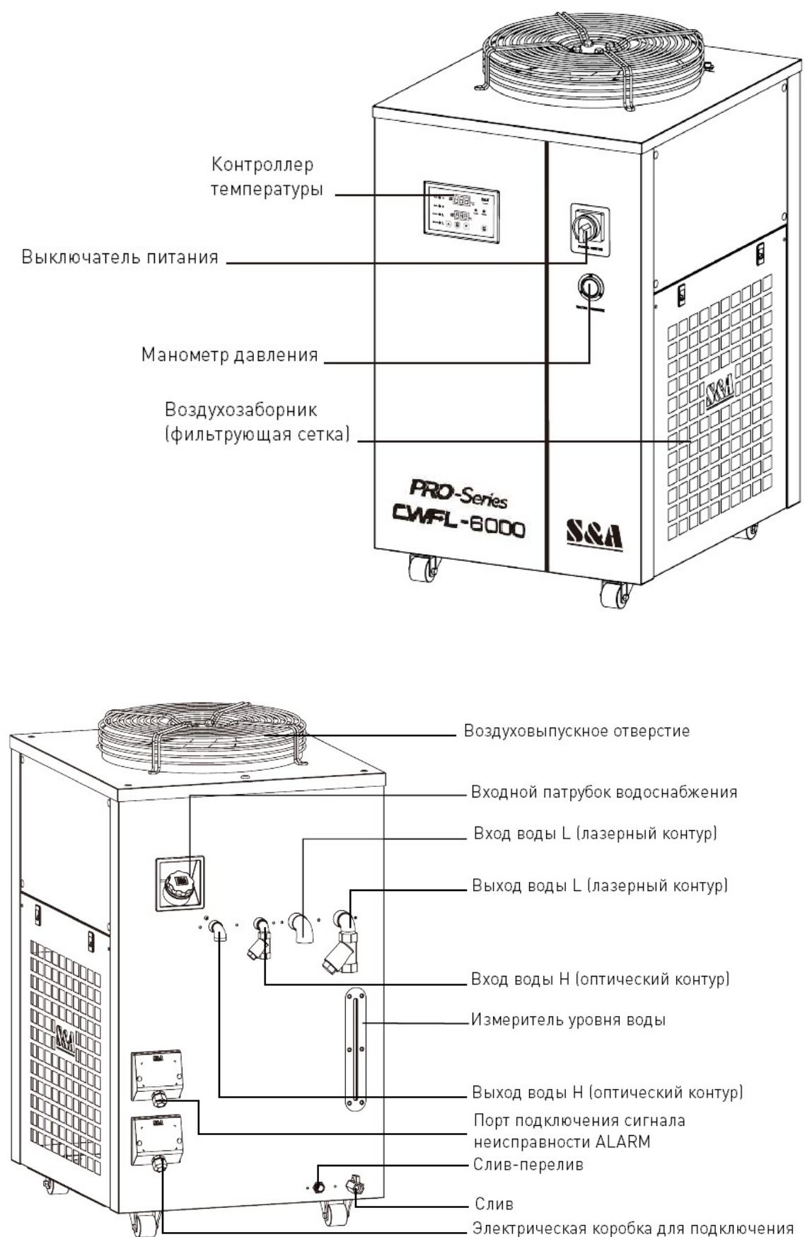
Рисунок 1 – Элементы чиллеров для лазеров от 1 до 6 кВт.
