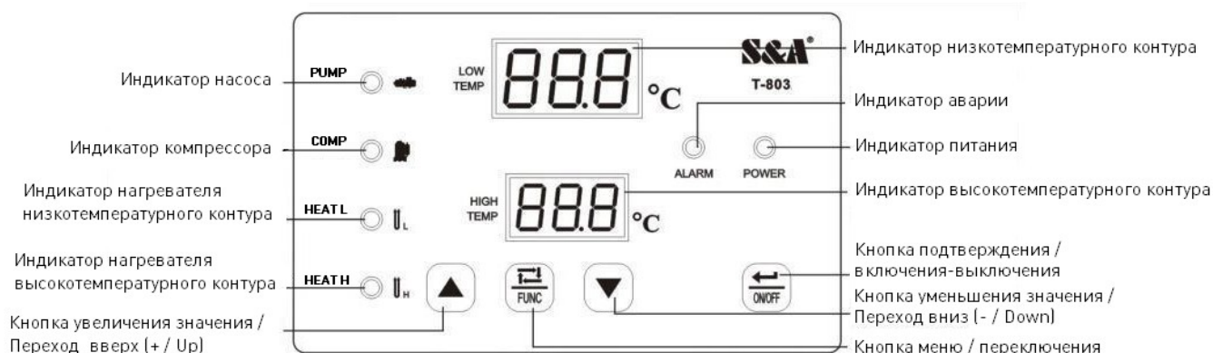
Рисунок 5 – Панель контроллера температуры.
