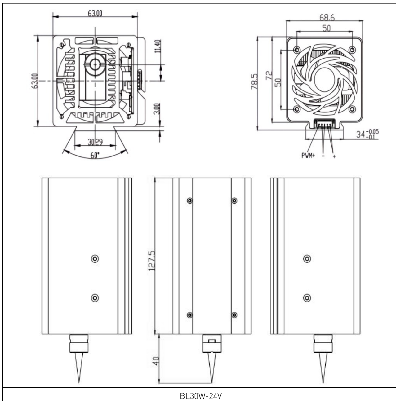
Рисунок 2 – Габаритные чертежи с указанием клемм подключения.
