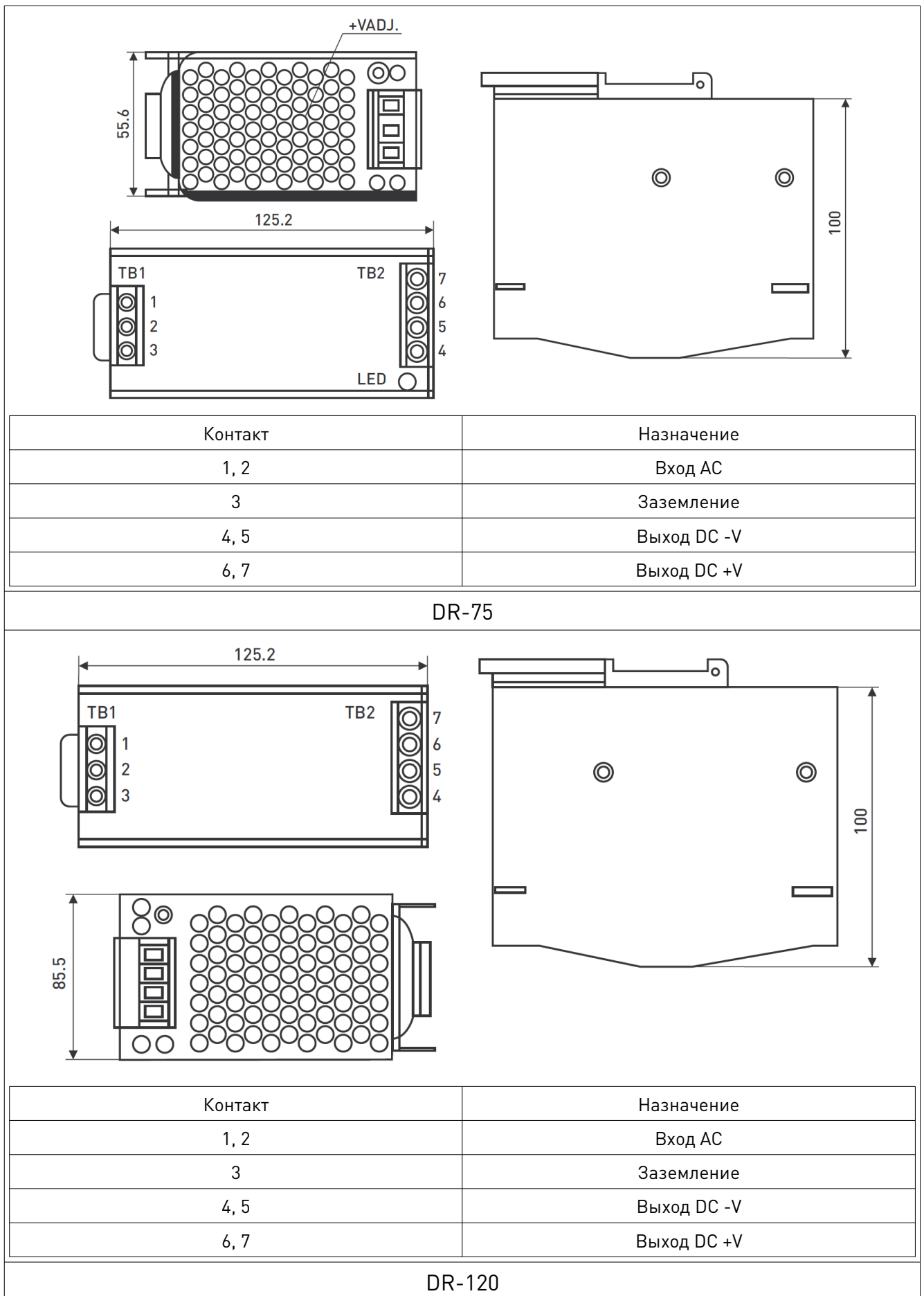
Рис. 2. Габаритные и установочные размеры источников питания
