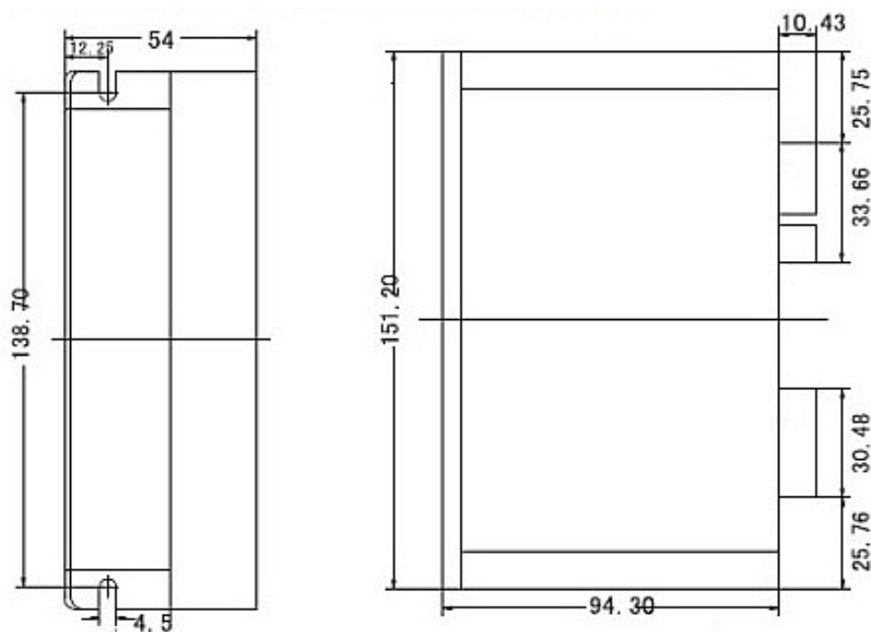
Рис. 1. Внешний вид драйвера
