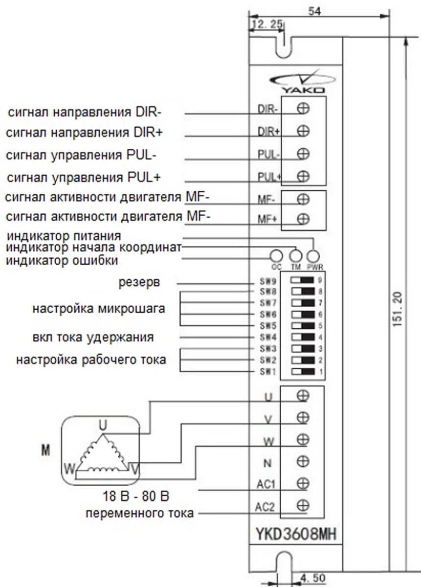
Рис. 3. Подключение драйвера
