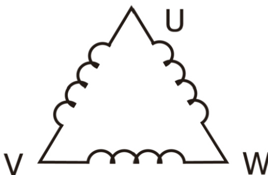
Рис. 5. Схема подключения шагового двигателя
