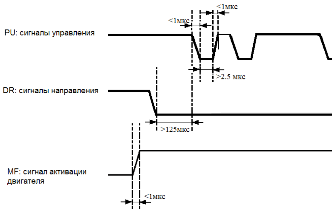
Рис. 4. Схема последовательности управляющих сигналов
