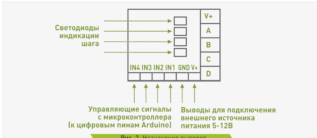
Рис. 2. Назначение выводов
