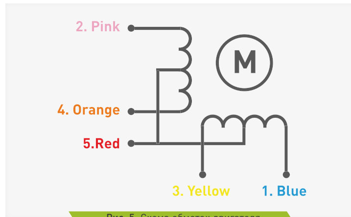
Рис. 5. Схема обмоток двигателя
